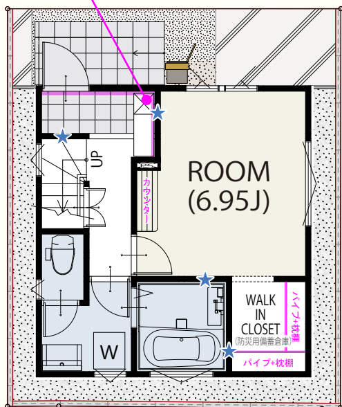
1 FLOOR / 28.14㎡ (防災用備蓄倉庫2.75㎡含む)
